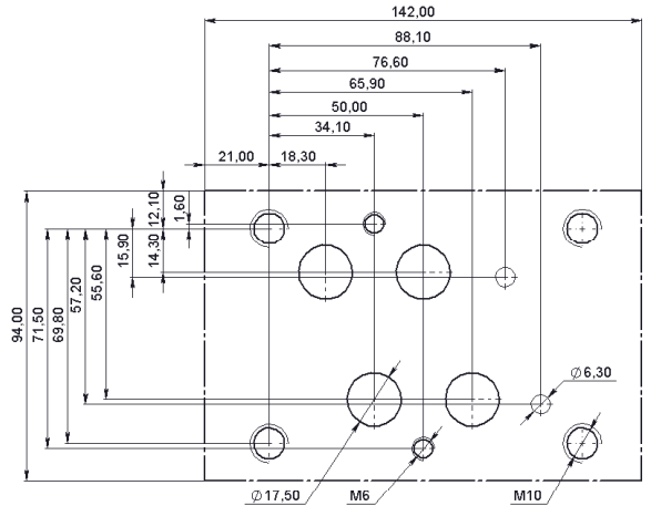
Монтажна плита Ду 16 Mounting plate NG 16
