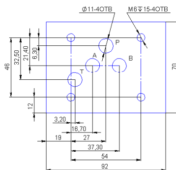
Монтажна плита Ду 10 Mounting plate NG 10
